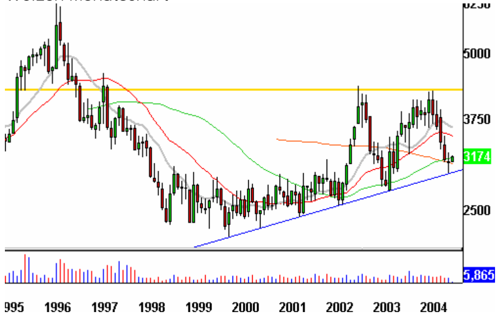
Weizen Monatschart
