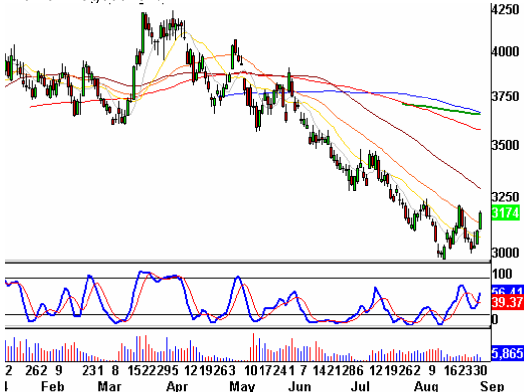
Weizen Tageschart
