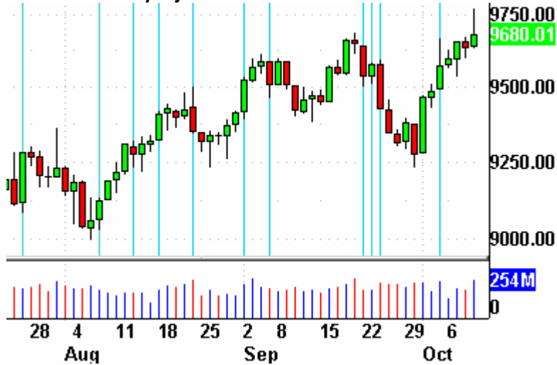
Dow Jones Zeitprojektionschart
